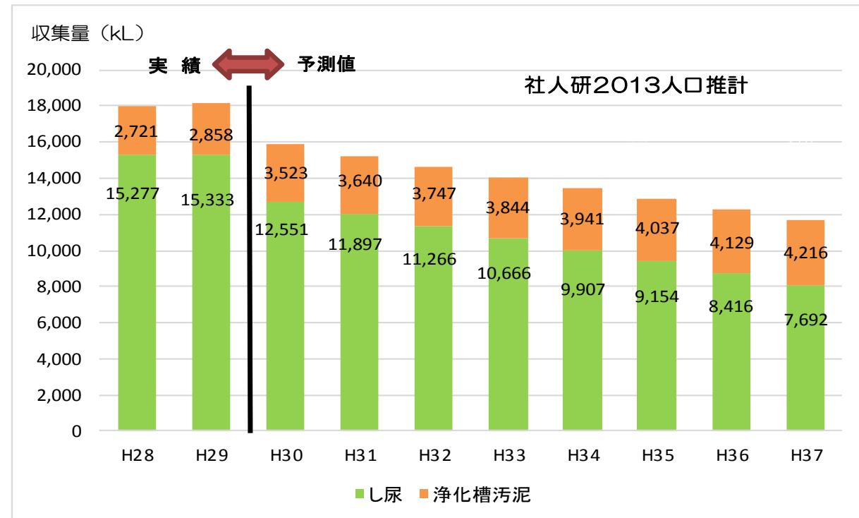
図5.1 し尿・浄化槽汚泥収集量の見込み（当初計画値）
